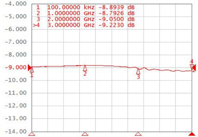
图2.插入损耗
